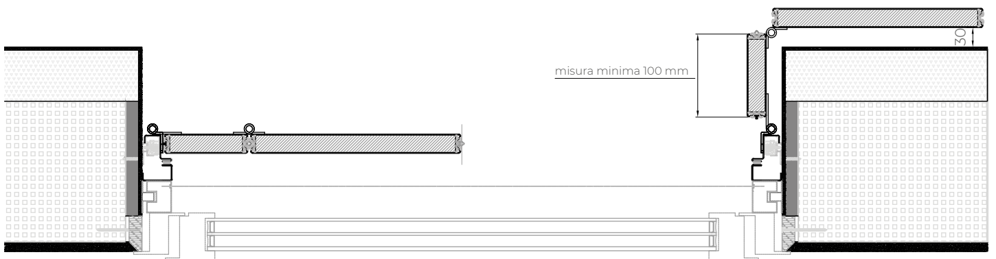
Sezione anta chiusa
